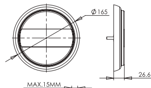
WIDOK WERSJI Z OZDOBNYM PIERSCIENIEM VIEW OF THE VERSION WITH DECORATING RING
