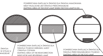
OGRANICZENIA W MONTAŻU LAMP JAKO ZESPÓŁ DWÓCH ŚWIETEL NIEZALEŻNYCH
