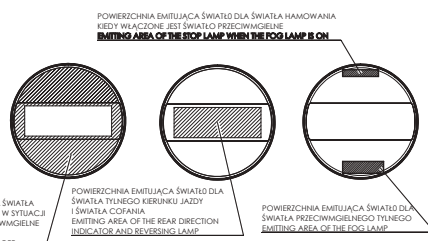
OGRAZNIENIA W MONTAŻU LAMP JAKO ZESPÓŁ DWOCH ŚWIATEŁ NIEZALEŻNYCH RESTRICTIONS ON THE LAMP ASSEMBLY AS A SET OF TWO INDEPENDENT LAMPS
