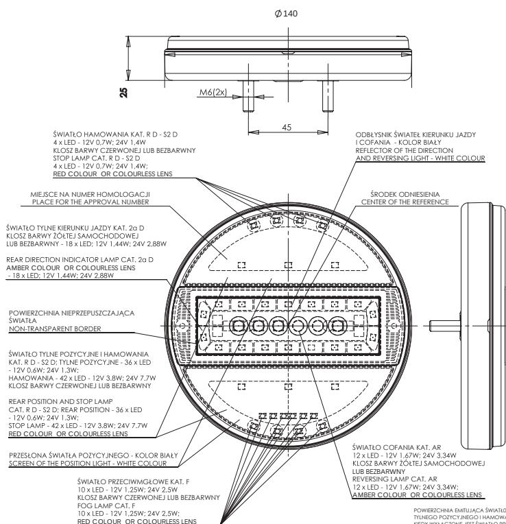
OGRAZNIENIA W MONTAŻU LAMP JAKO ZESPÓŁ DWOCH ŚWIATEŁ NIEZALEŻNYCH RESTRICTIONS ON THE LAMP ASSEMBLY AS A SET OF TWO INDEPENDENT LAMPS
