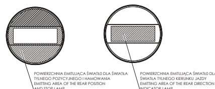
OGRODNICZENIA W MONTAŻU LAMP JAKO ZESPÓŁ DWAÓCH ŚWIATEŁ NIEZALEŻNYCH RESTRICTIONS ON THE LAMP ASSEMBLY AS A SET OF TWO INDEPENDENT LAMPS
