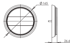
WIDOK WERSJI Z OZDOBNYM PIERŚCIENIEM VIEW OF THE VERSION WITH DECORATING RING
